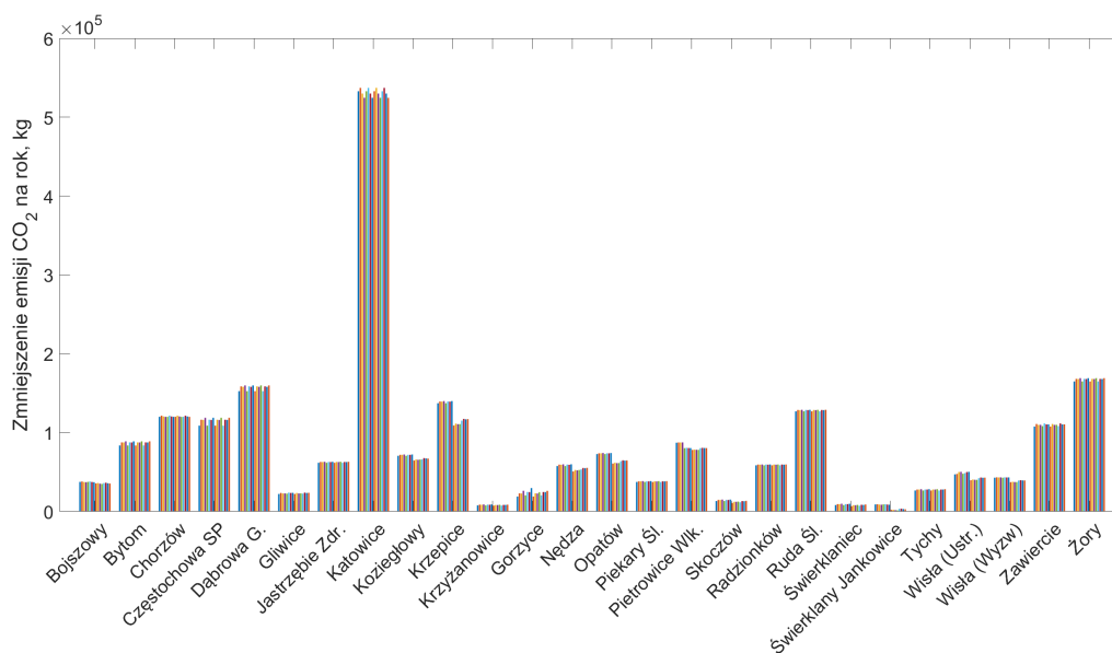
Rysunek 7: Roczna, uniknięta emisja CO 2 dla poszczególnych wariantów obliczeniowych.
