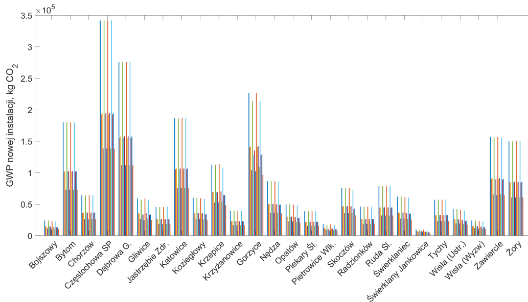
Rysunek 8: Ekwiwalent CO 2 związany z budową instalacji dla poszczególnych wariantów obliczeniowych.
