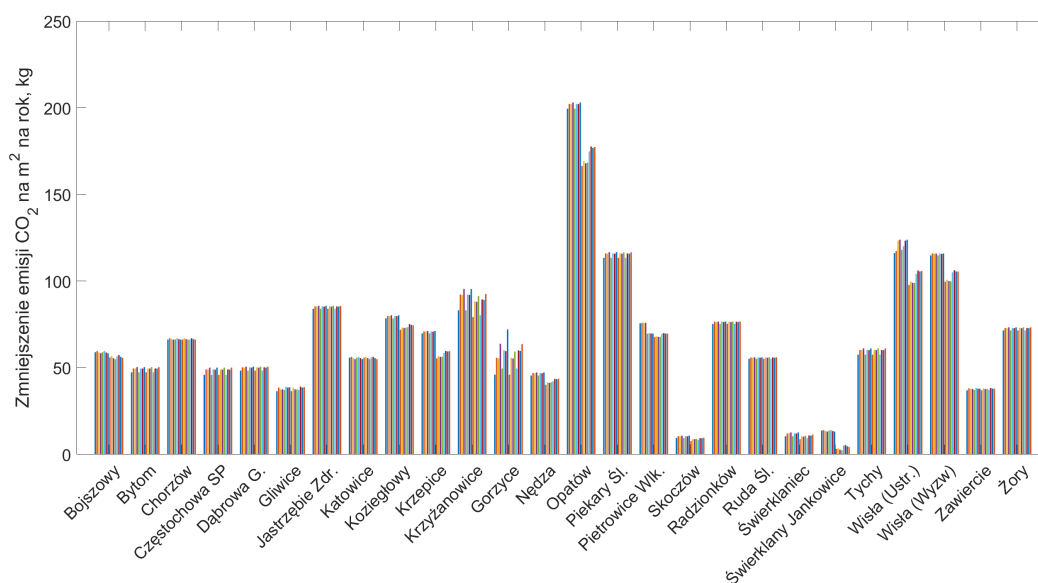
Rysunek 6: Względna (w odniesieniu do jednostki powierzchni), roczna, uniknięta emisja CO 2 dla poszczególnych wariantów obliczeniowych.
