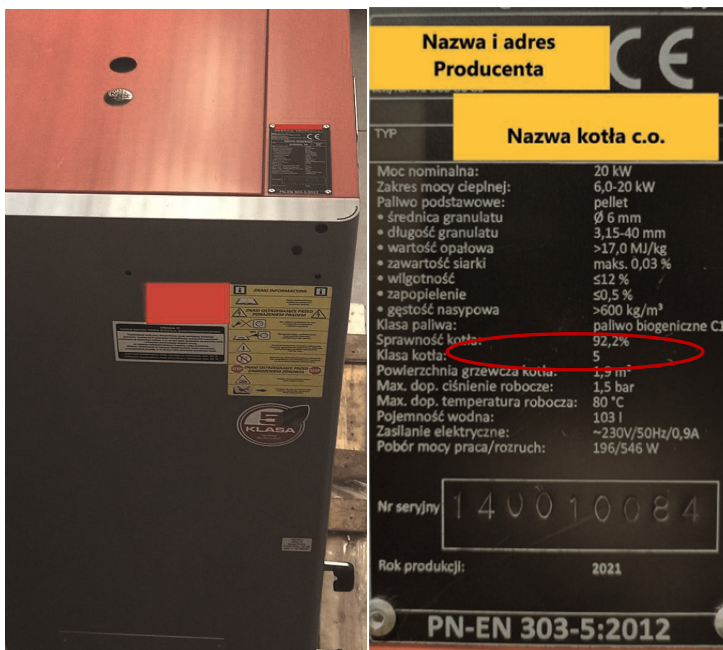
Rys. 8. Tabliczka znamionowa kotła
