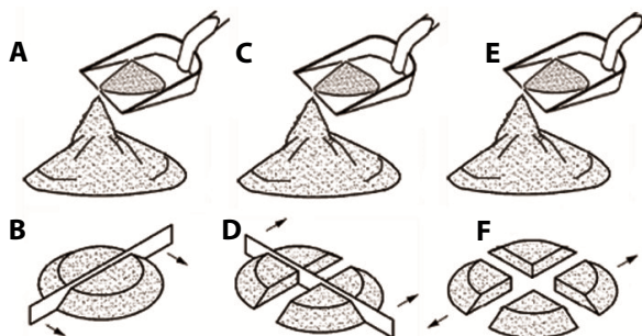
Rys. 13. Sposób pobierania próbki odpadu paleniskowego metodą kwartowania
